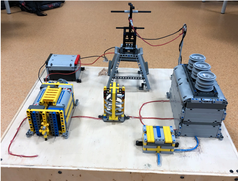
CENTRALE GEOTERMICA
